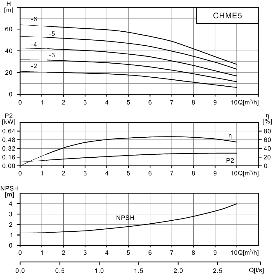
CHME5性能表
