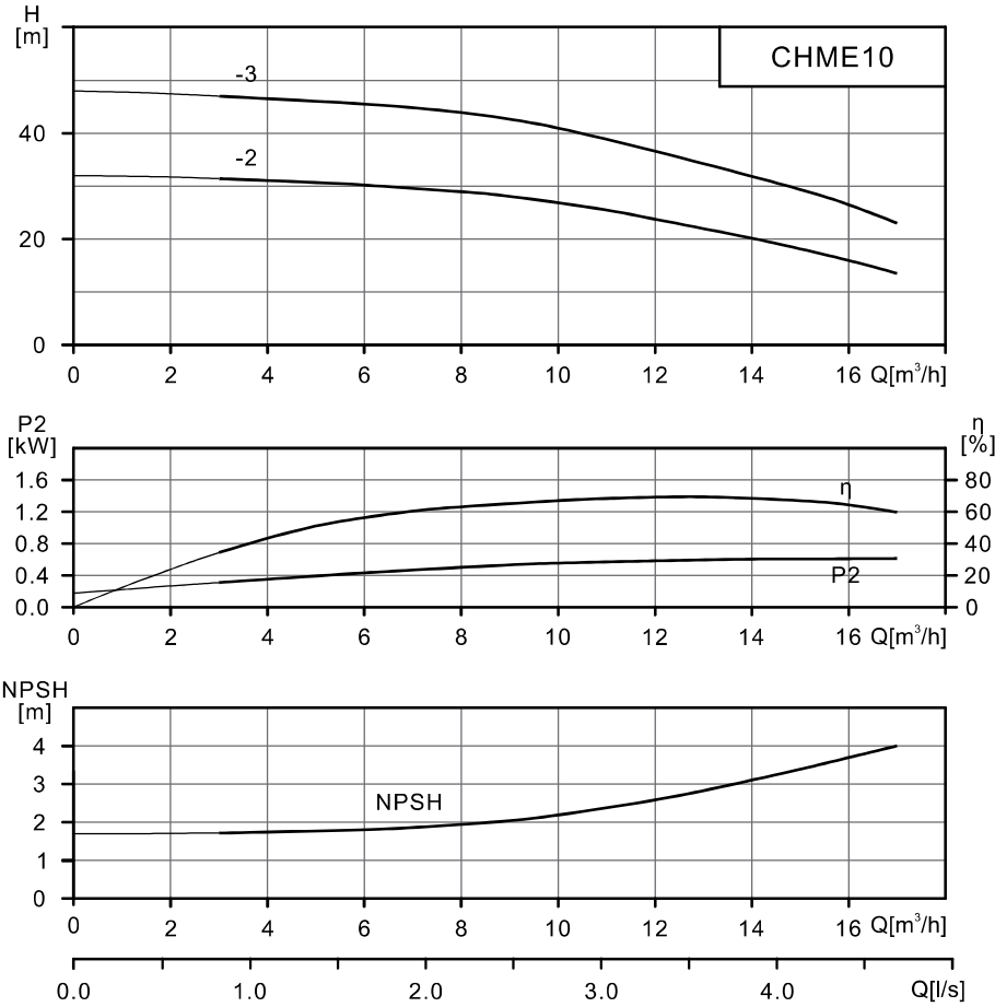
CHME10性能表
