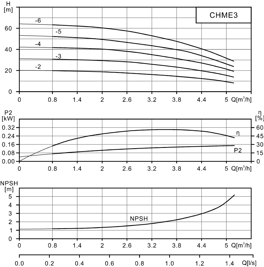
CHME3性能表
