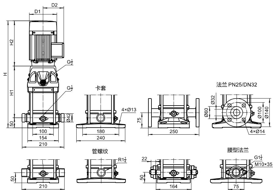
LDMF5 安装尺寸图
