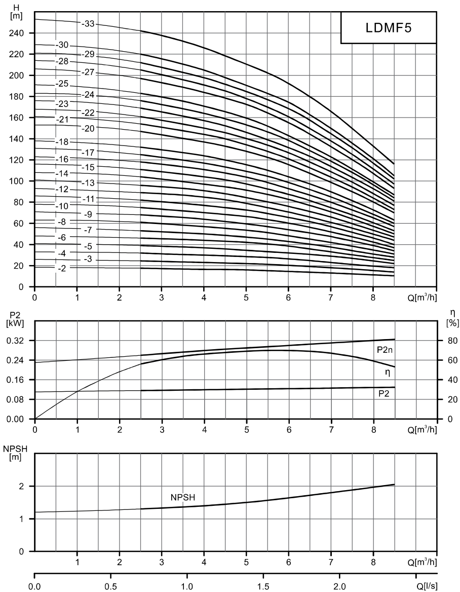
LDMF5 性能曲线
