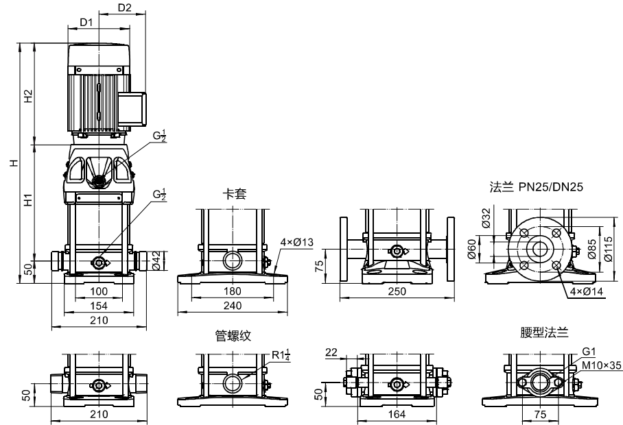
LDMF3 安装尺寸图
