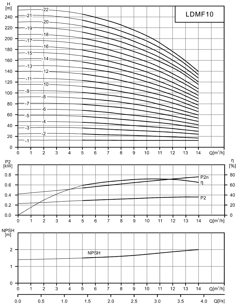
LDMF10 性能曲线
