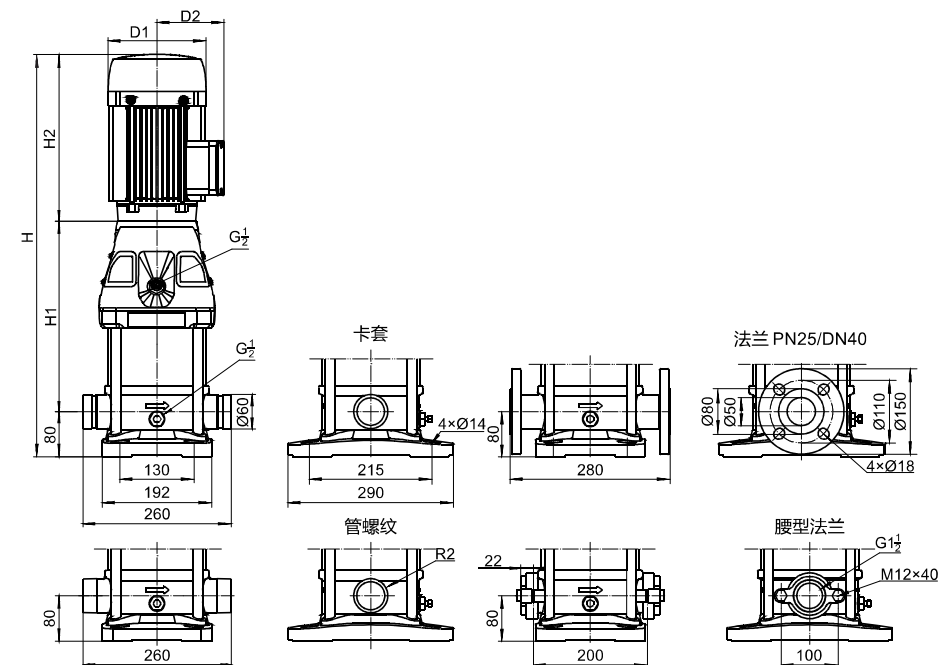
LDMF10 安装尺寸图
